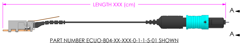
PART NUMBER ECUO-B04-XX-XXX-0-1-1-5-01 SHOWN
