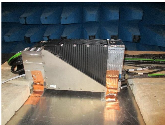
Vue générale de l'Équipement Sous Test (E.S.T)
