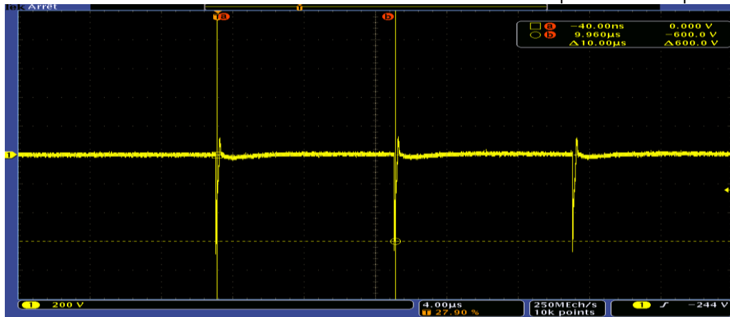
Répétition entre 2 spikes
