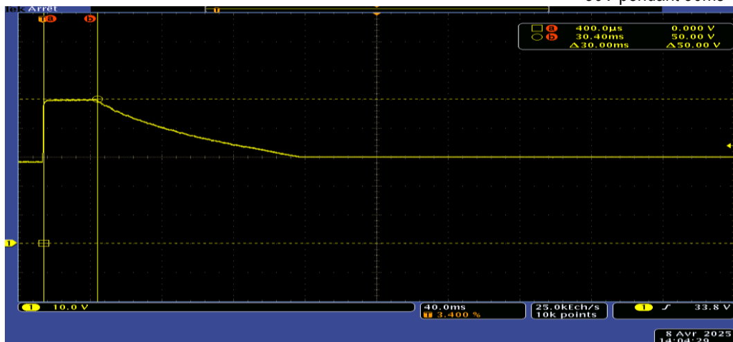
Courbe 3 50V pendant 30ms
