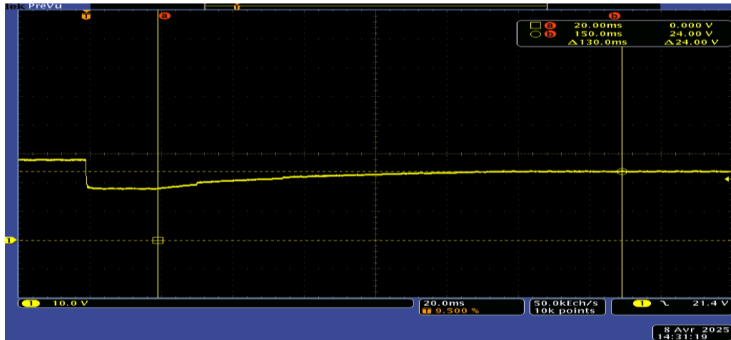
Courbe 6 18V à 24V en 130ms
