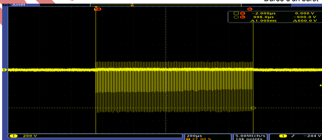
Durée d'un burst
