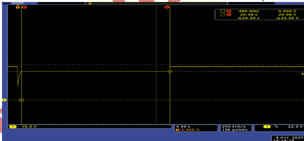
Courbe 4 24V pendant 20s
