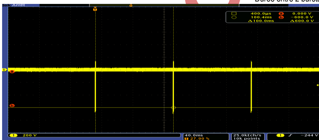
Durée entre 2 bursts
